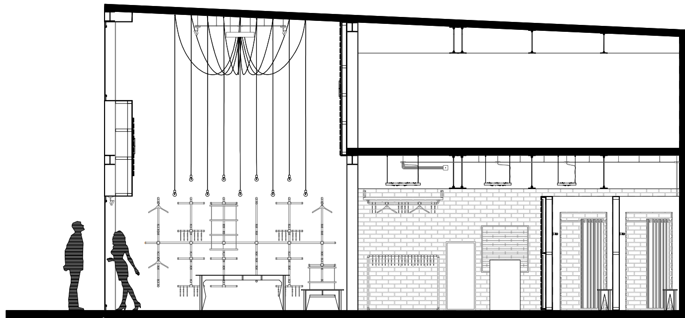
Elevación Sur
