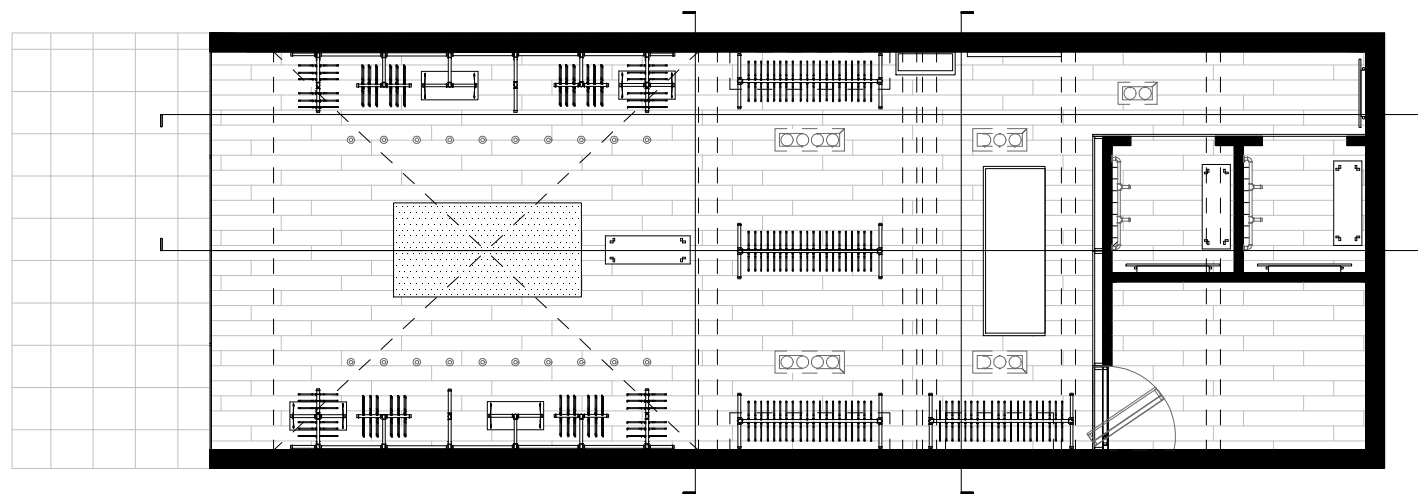
Planta
